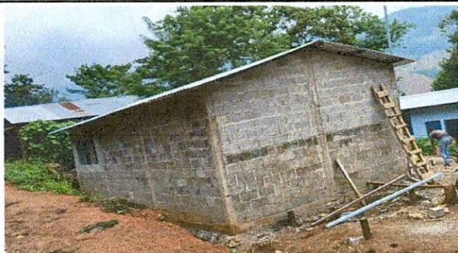
Foto: 5 INSTALACIÓN DE TECHO Y CUBIERTA DE LAMINA MÓDULO 2
